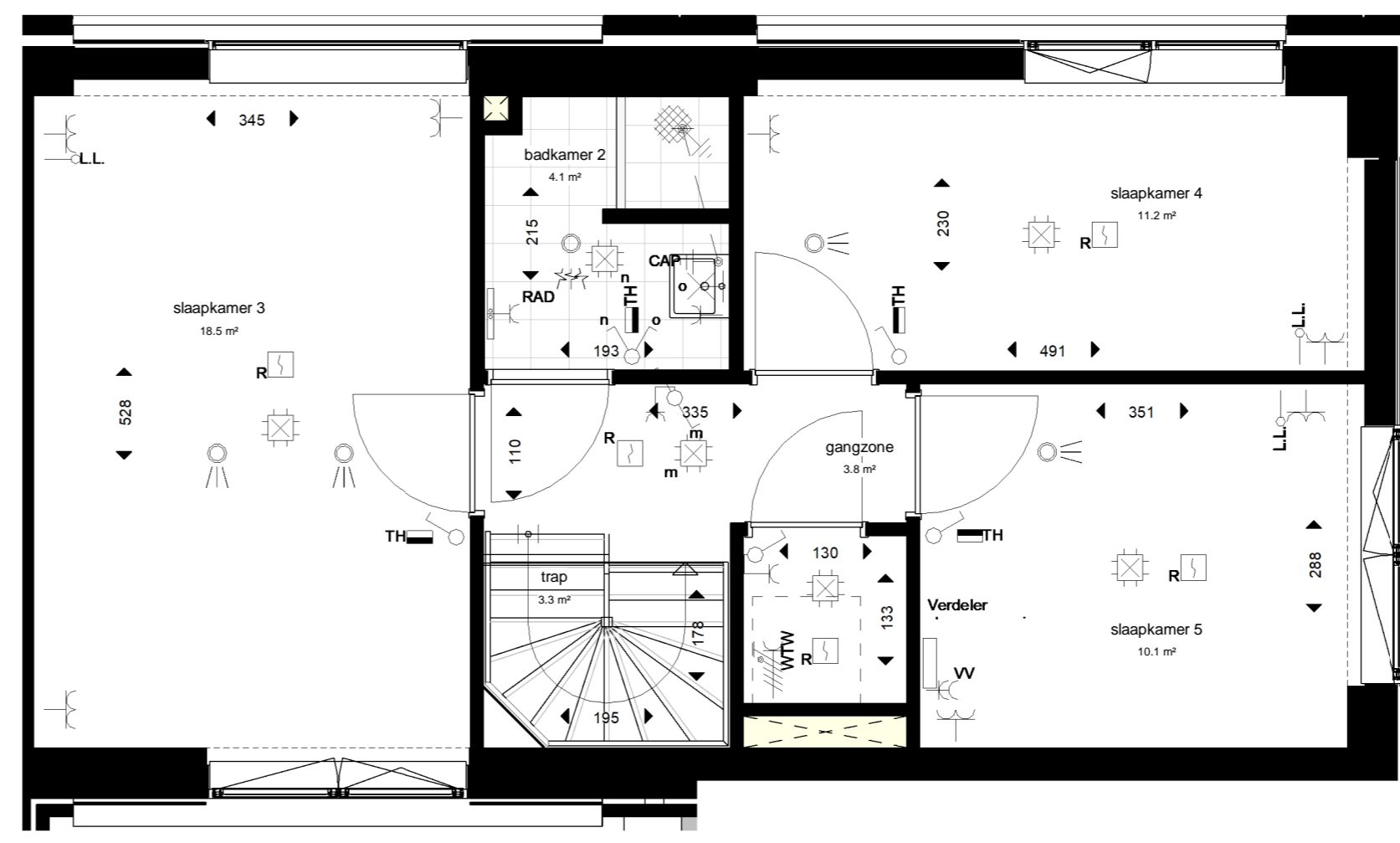
3e verdieping
