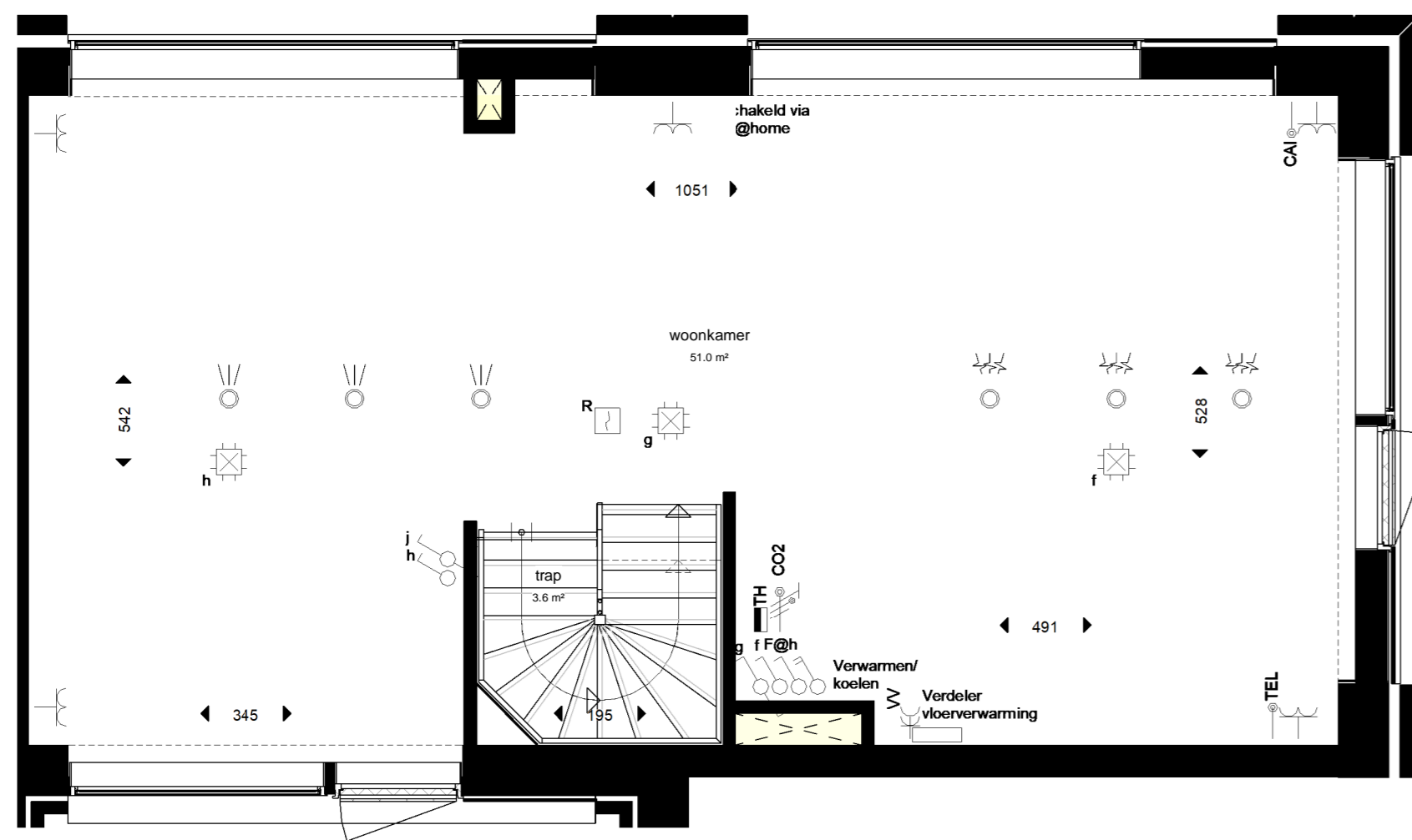
1e verdieping
