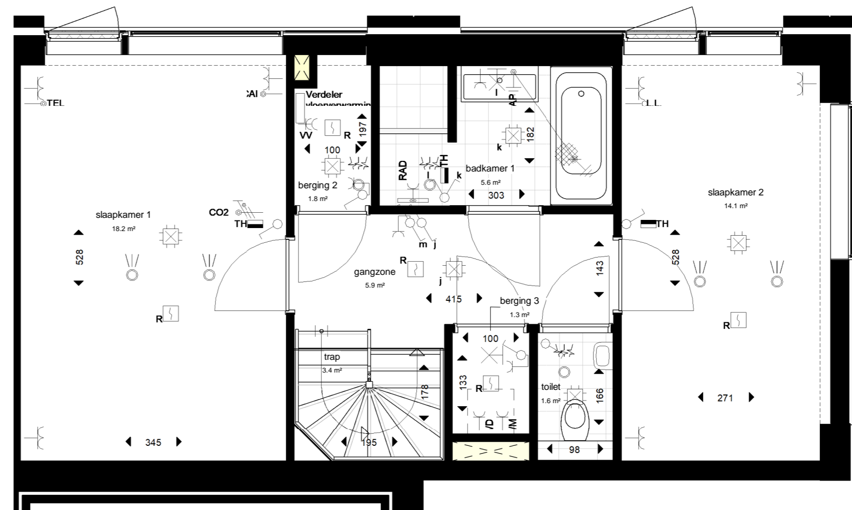
2e verdieping
