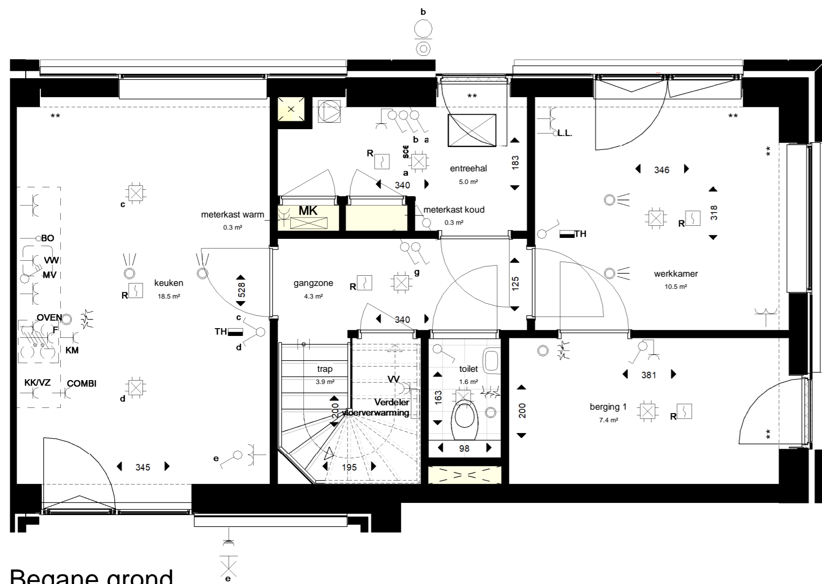
Begane grond
